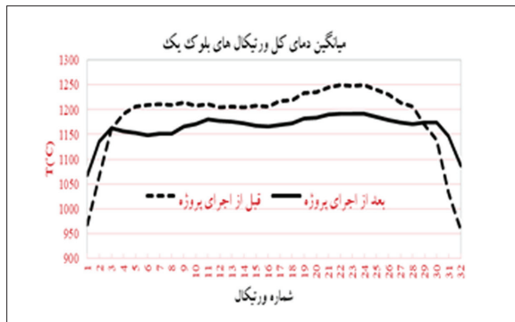
شکل شماره ۱: دمای و ریتیکال های کل باطری در بلوک ۱ و ۲ قبل و بعد از اجرای پروژه
